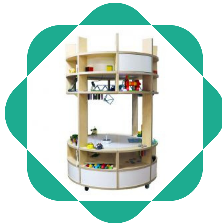
I VULCANI
